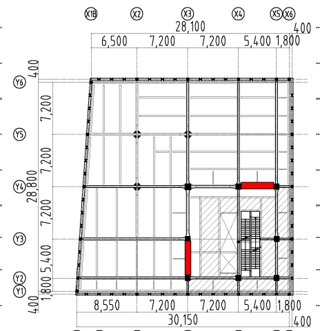
基準階(5階)伏図
