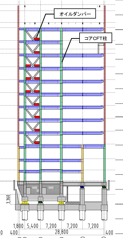
X3軸組図
