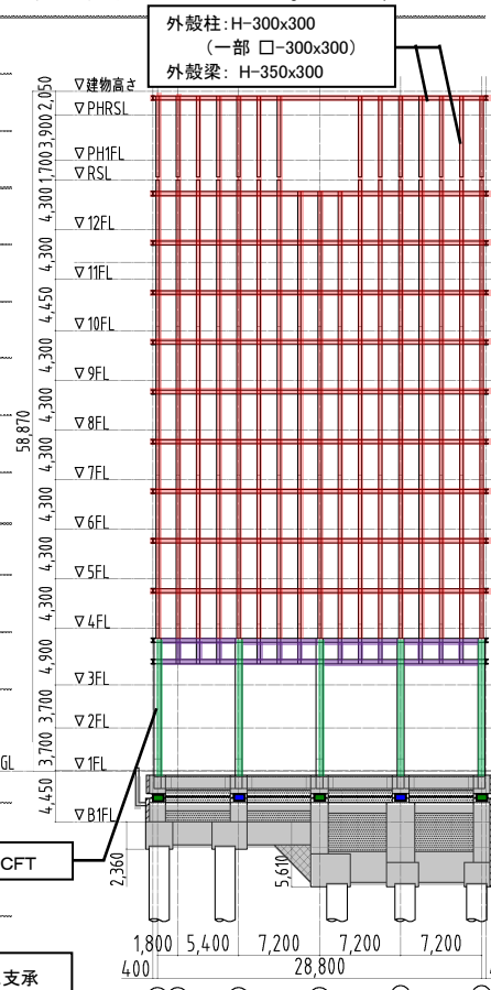
X1A-X1B軸組図
